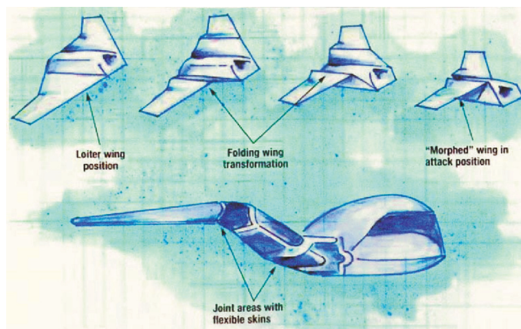
Slika 10. Mogućnost promjene oblika krila zrakoplova u letu kao primjer kontrolirane prilagodbe konstrukcije u više točaka
