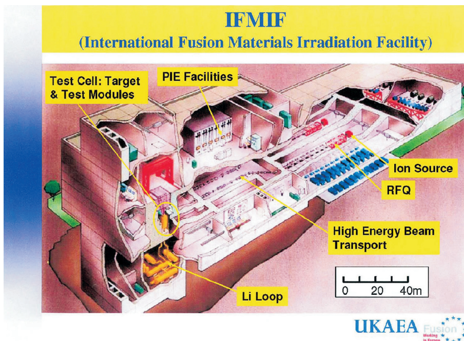
Slika 14. Postrojenje za ispitivanje izdržljivosti materijala za izgradnju fuzijskog nuklearnog reaktora
