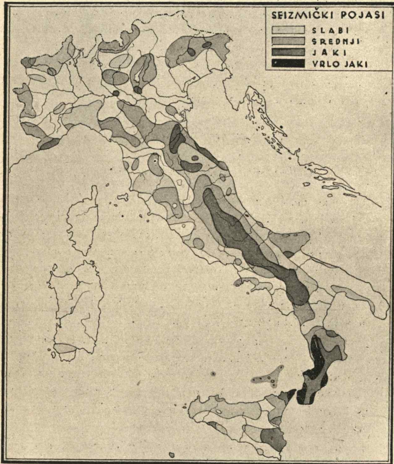
Slika 2. Seizmički pojasi (A. Gortani)
