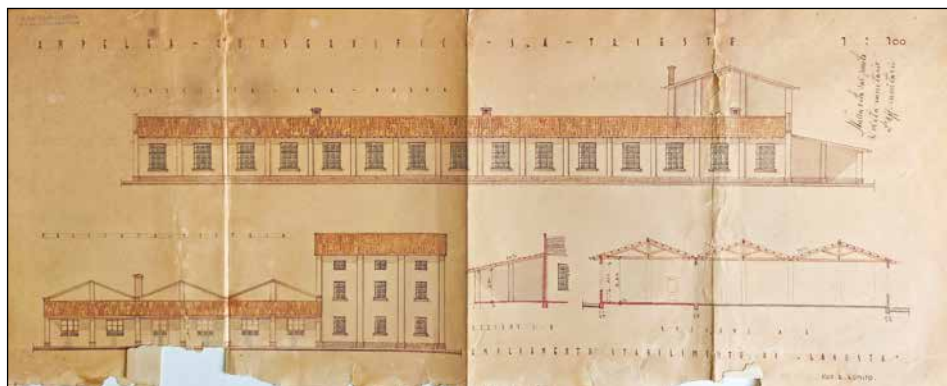
Slika 5. Projekt proširenja tvornice za preradu ribe u Ublima: pogledi i presjeci, autor: R. Romito, bez godine (HR-DADU-SCKL-732. Općina Lastovo).
