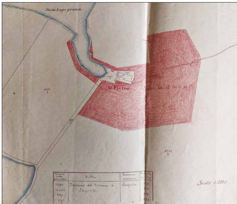
Slika 2: Situacijski nacrt tvornice u Ublima, bez oznake autora i godine. Površina od oko 22 ha označena crvenom bojom oko tvornice možda predstavlja širi obuhvat koji je uzet u obzir za daljnu regulaciju ovog područja, no ona je znatno veća od površine tvornice i naselja. (HR-DADU-SCKL-732. Općina Lastovo).
